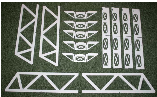
*Teileübersicht 850mm Version
